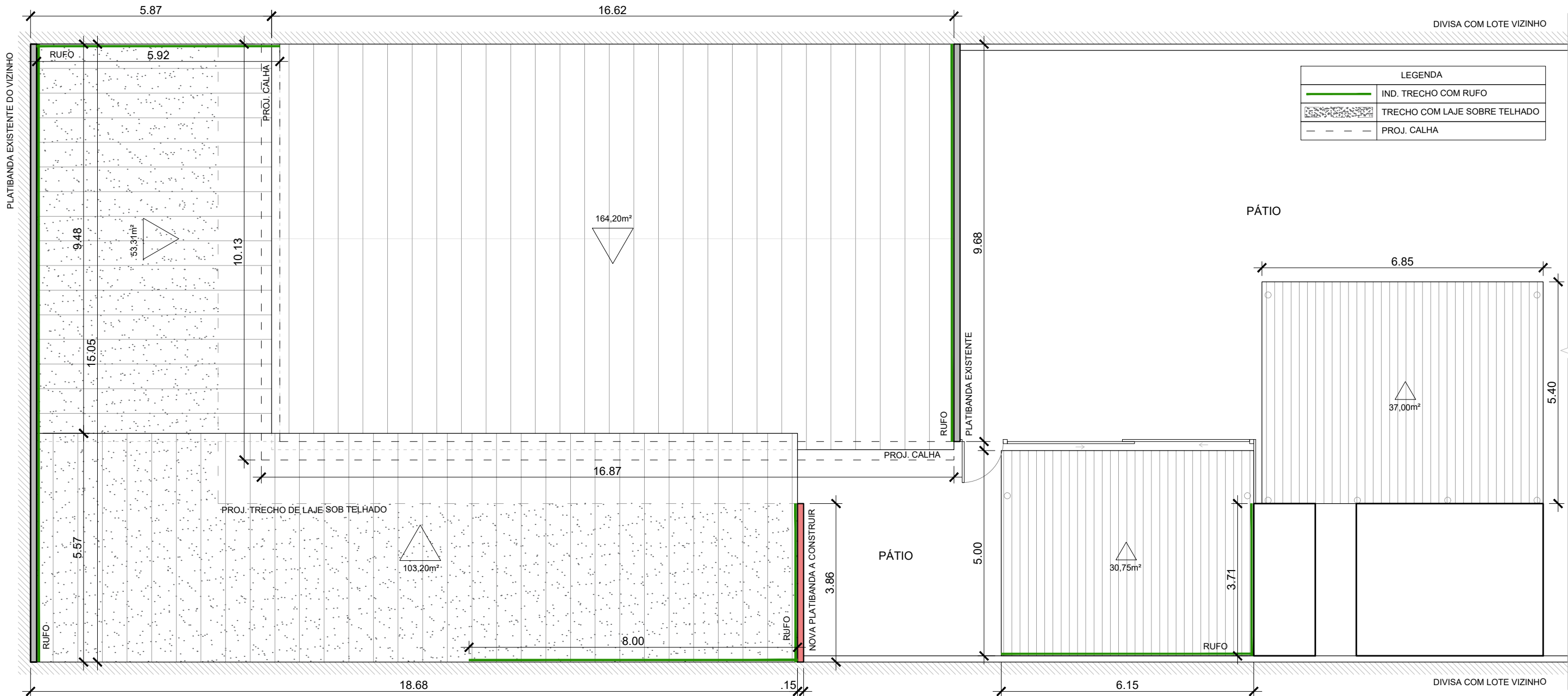
1 PLANTA ESQUEMÁTICA DE COBERTURA ESC.: 1/100
