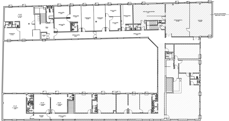
2 PLANTA DE ARQUITETURA - 2º PAV ESC.: 1:250
