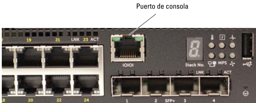
Ilustración 1-9. Panel frontal de N1524P con puerto de consola
